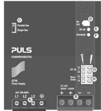
Fig. 15-1 Front side
