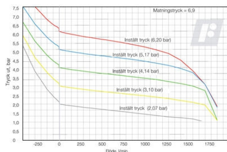
Flödeskurva 10262
