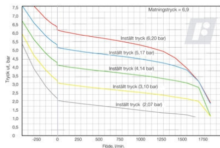
Flödeskurva 10262
