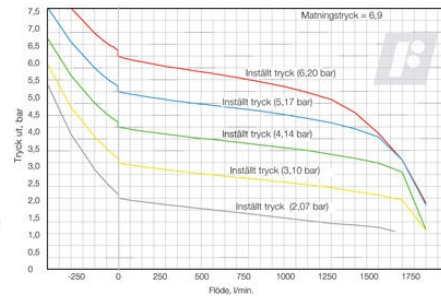
Flödeskurva 10262
